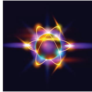
Neutrino-deeltje
